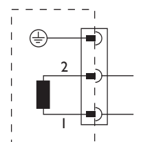
DIN 43650-1 Form A: 2+PE - PG9
